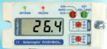
Differenztemperaturregelgerät
