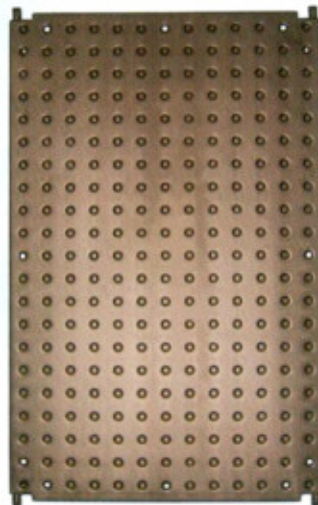
Art.-Nr. 1001 mit 4 Anschlußstutzen Ø 25 mm Länge 1.280 mm - Breite 820 mm - 1.05 m 2
