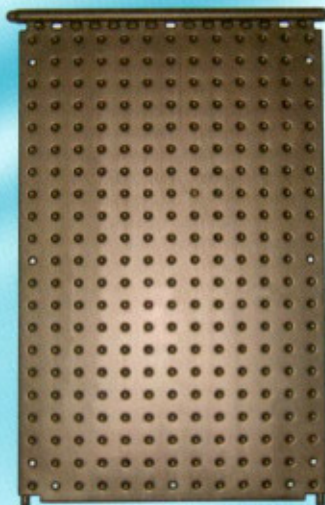
Art.-Nr. 1000 mit integriertem Sammelrohr Ø 40 mm und 2 Anschlußstutzen Ø 25 mm Länge 1.320 mm - Breite 820 mm - 1.08 m 2
